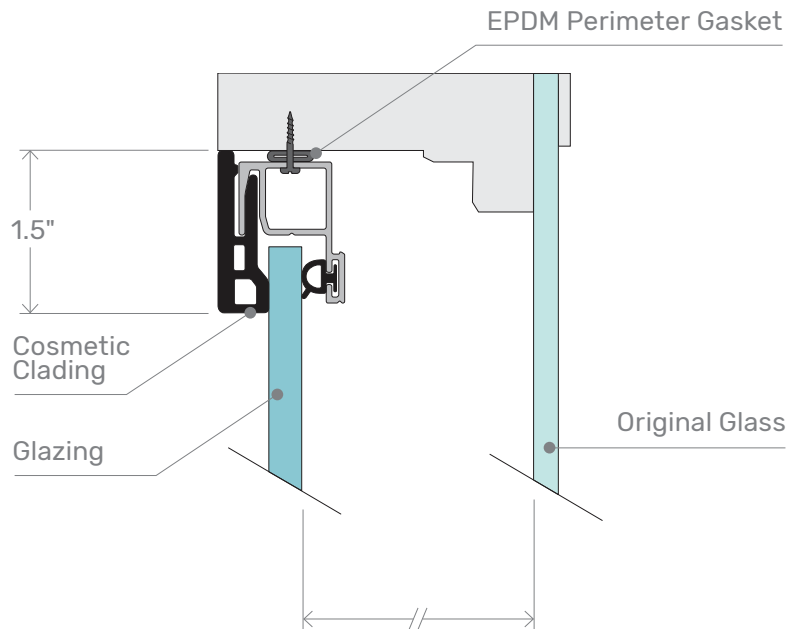
C Jamb Detail
